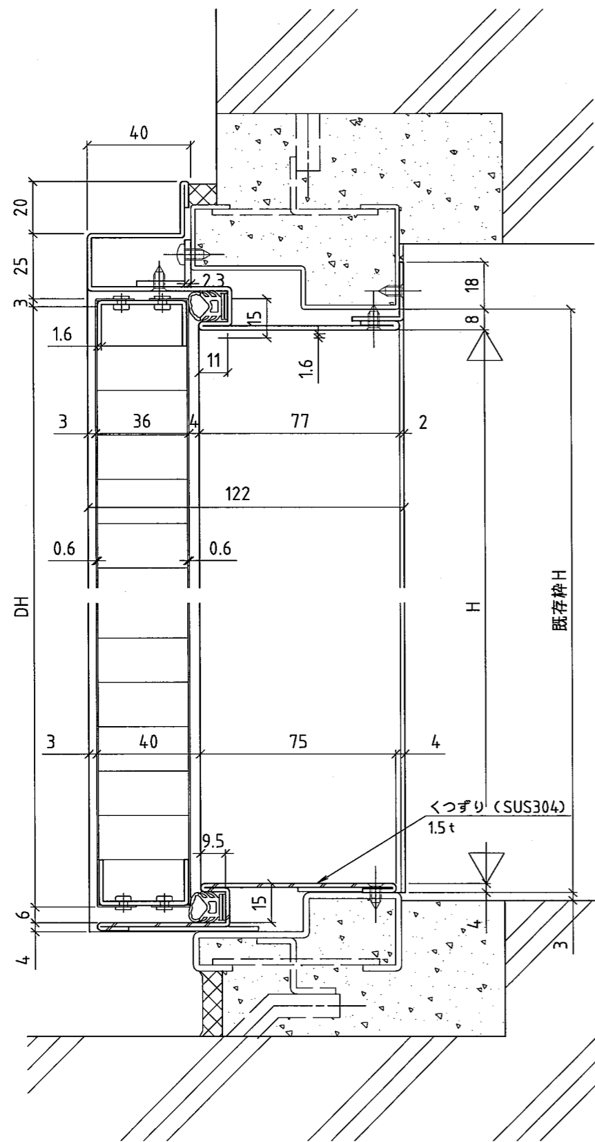
< 垂直断面図 >
