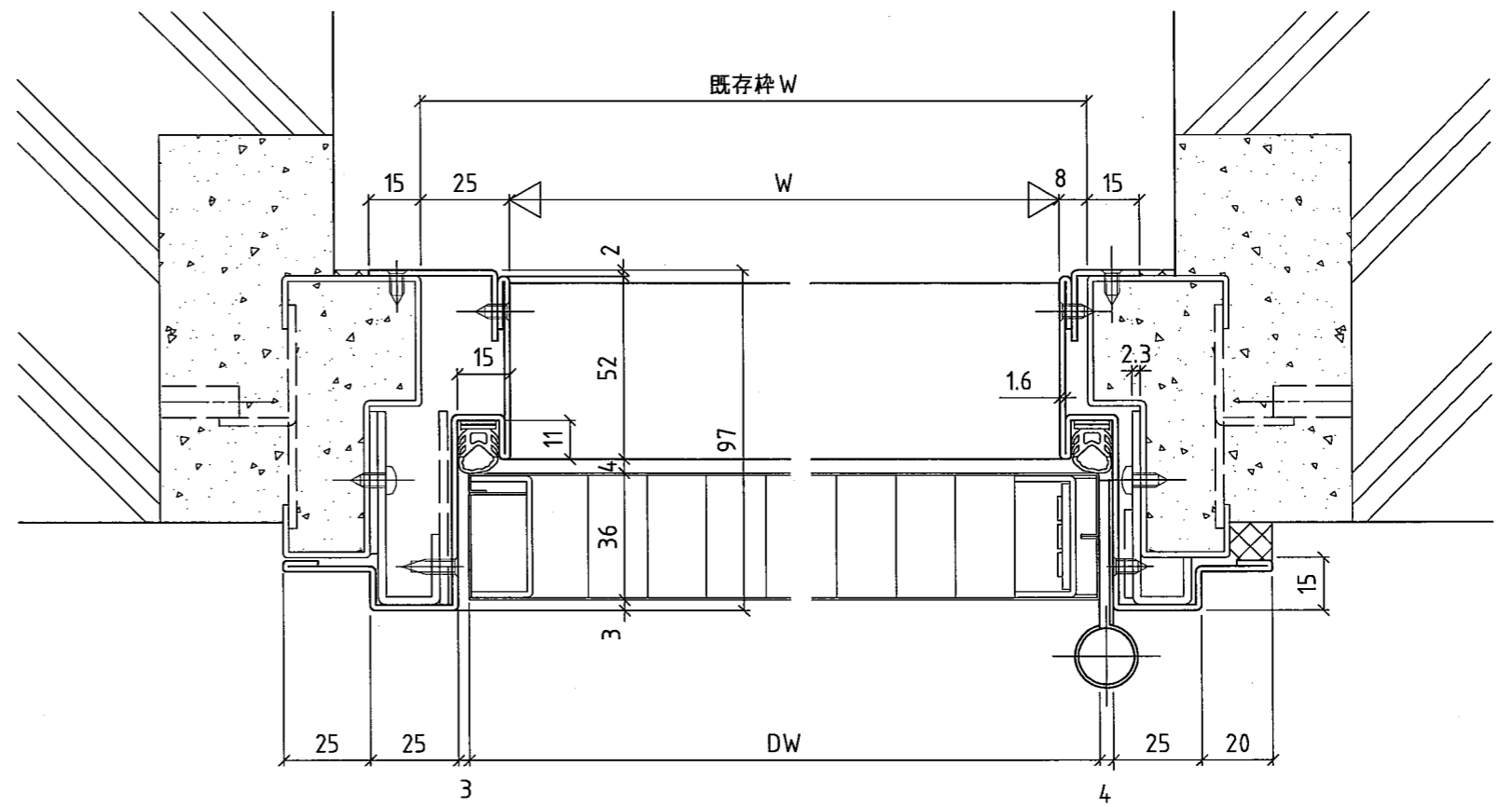
<水平断面図>
