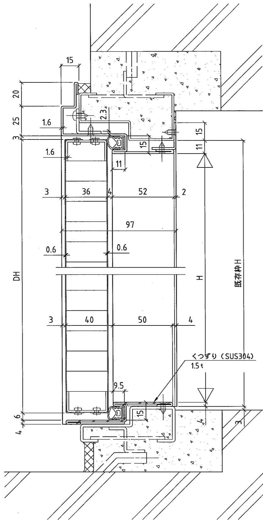
<垂直断面図>
