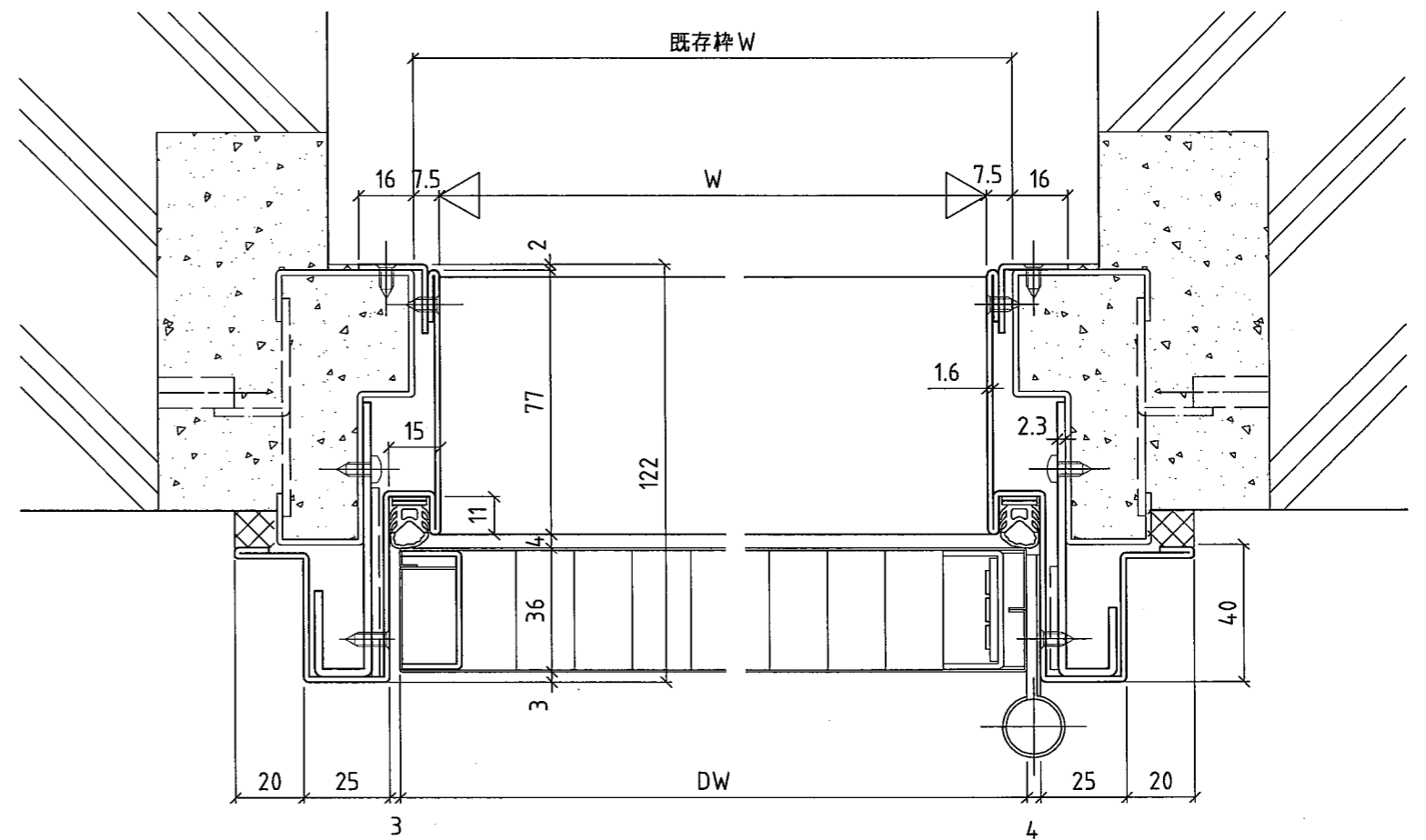
< 水平断面図 >
